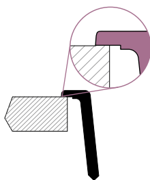
Horní uložení montáž bez příchytek
