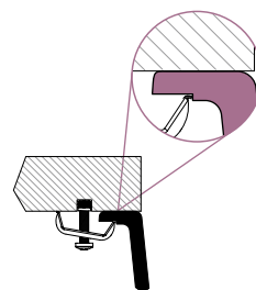
Spodní uložení montáž s příchytkami
