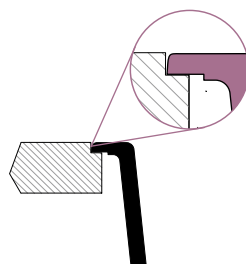
Uložení do roviny montáž bez příchytek
